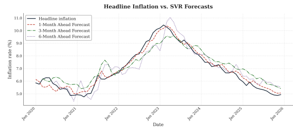
(d) SVR
